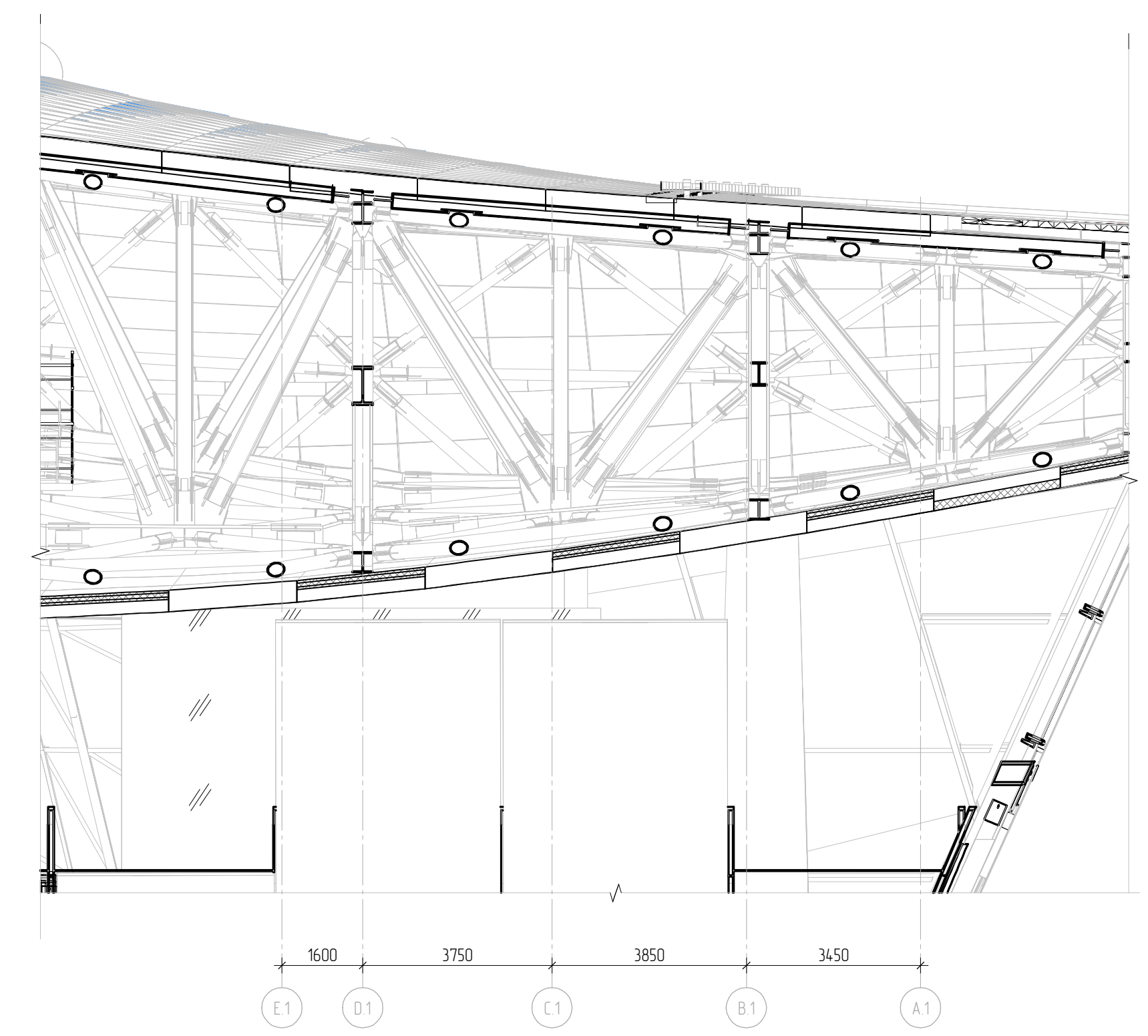
Сечение Ж-Ж (1 : 100 )
